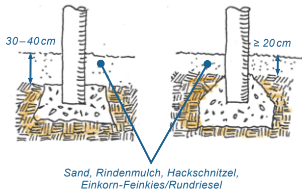
Mindestbodenüberdeckungen von Fundamenten
